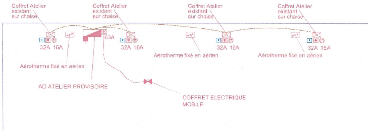
ATELIER PROVISOIRE Atelier énergie voie 120m 2
